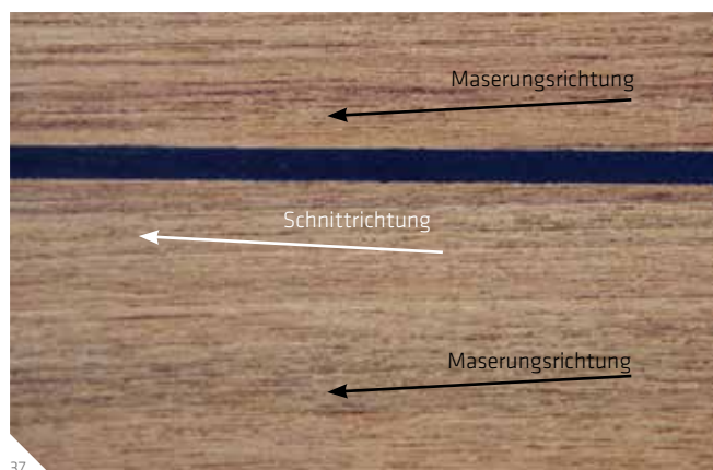
37 Die Schneiderichtung sollte mit der Maserung verlaufen, um Abschürfungen an den Stabdeckleisten zu verhindern.
