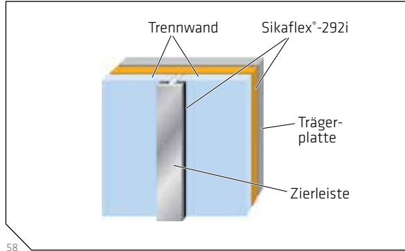
58 Abb. 58: Sikaflex®-292i Applikation
