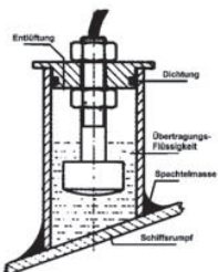
7370 Inneneinbausatz für Echolotswinger N40 Befestigungsmutter (Wird bei Verwendung des Inneneinbausatzes benötigt)
